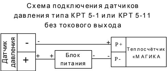
Схема подключения датчиков избыточного давления
