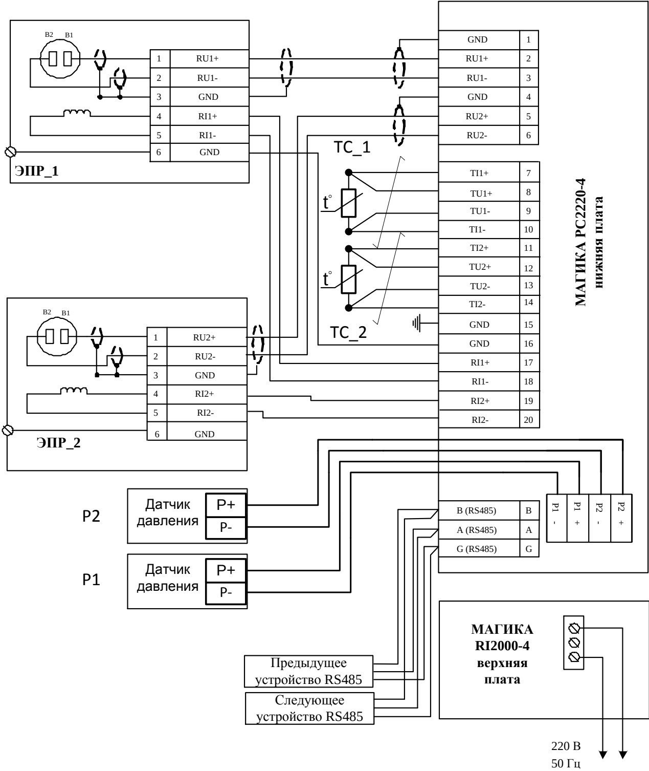
Схема подключения к ЭБ регистратора расхода электромагнитного «РС2220-4»
