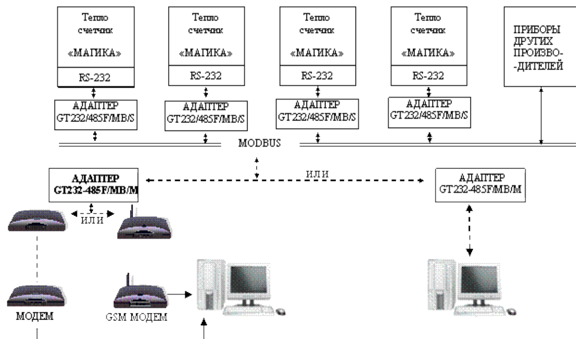
АДАПТЕР ИНТЕРФЕЙСА GT232F/Ethernet
